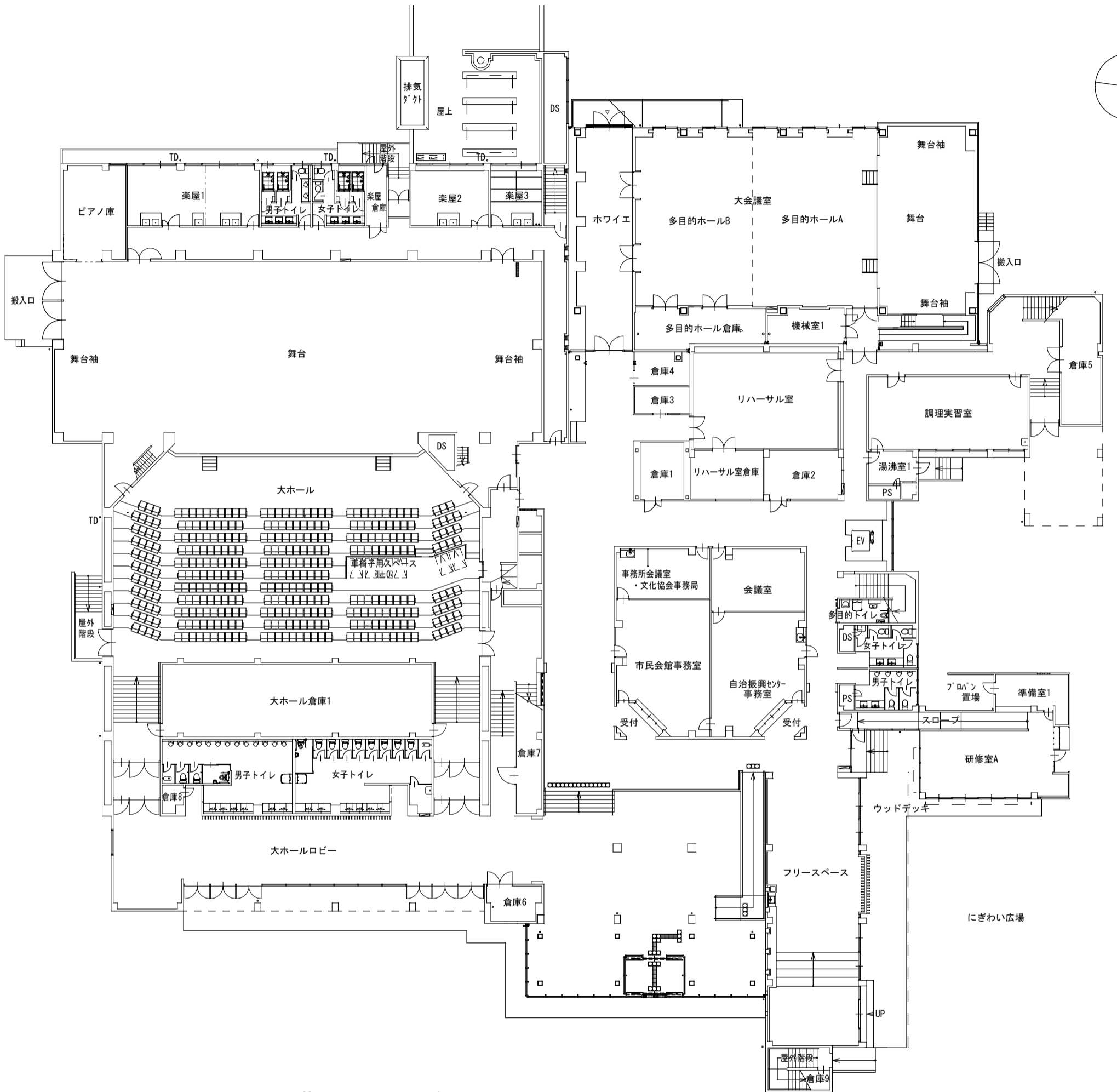
1階平面図 S=1/150
